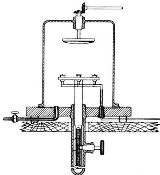
Vakuumkanter. Øverst hænger linsen, nedenunder ses en holder med små elektrisk opvarmede skåle som stoffet, der skal fordampes ligger i.
