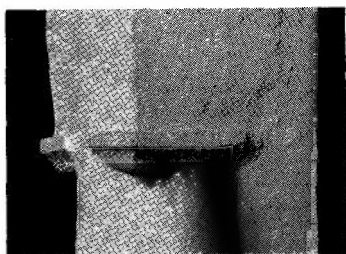
Fig. 2. Pille fra Tamdrup kirke. Ved hvælvingernes opførelse blev den oprindelig runde pille udvidet og forstærket.
