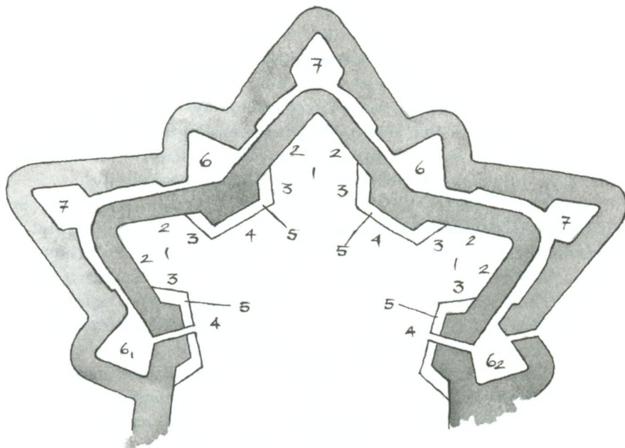
Skematisk oversigt over de fæstningsudtryk, der er nævnt i artiklen. 1: Bastion, 2: Face, 3: Flanke, 4: Kurtine, 5: Faussebrai, 6: Ravelin, 6 1 , 6 2 : Enveloppe, 7: Kontregarde. (Tegning: Christian Mosbæk Johannessen).
