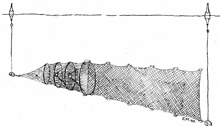
En Kasteruse (til Torsk). Tegn. af E. Mikkelsen.
