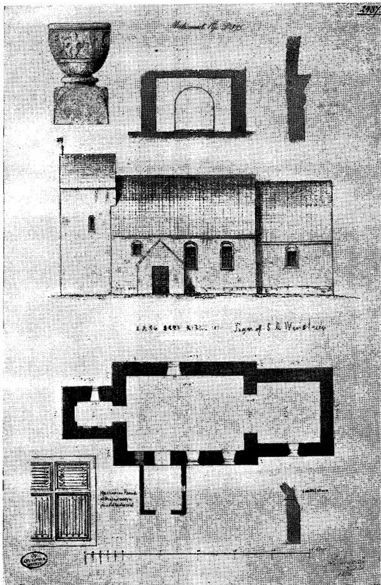
Øverst: Døbefont i Langskov Kirke (tegnet af S. A. Winstrup), — Snit af Langskov Kirkes Kor, — og: Profil af Korbuens Gesims I Midten: Langskov Kirke 1876 (tegnet af S. A. Winstrup). Nederst: Udskaaren Forside af Beklædningen paa Alterbordet, = Grundplan af Langskov Kirke, — og Profil af Sokkelsten.
