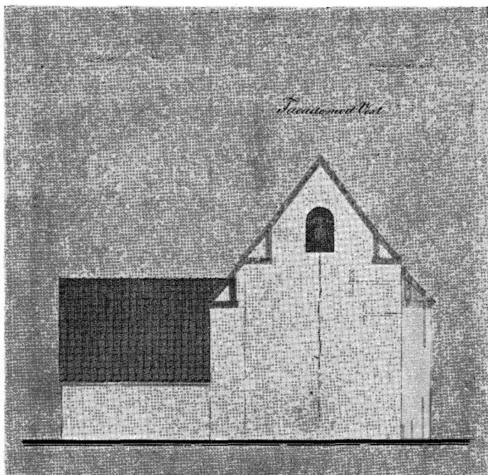
Uldum gamle Kirke, Facade mod Vest. Efter Tegn. i Nationalmuseet af Tage Olivarius.
