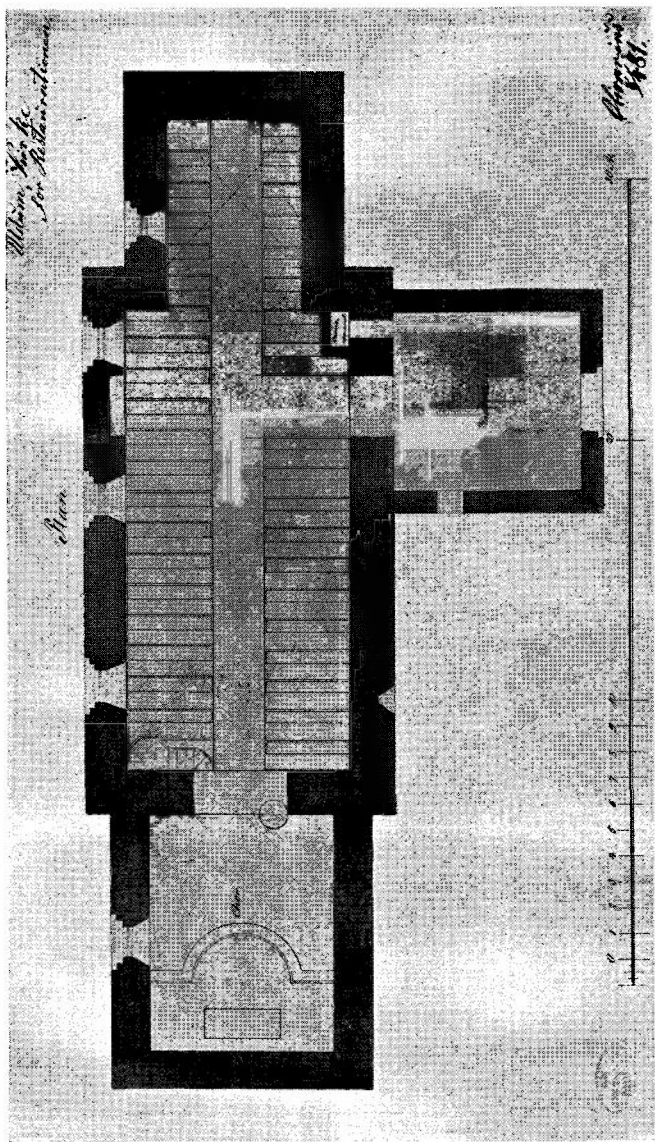
Uldum gamle Kirke, Grundplan. Efter Tegning i Nationalmuseet af Tage Olivarius.
