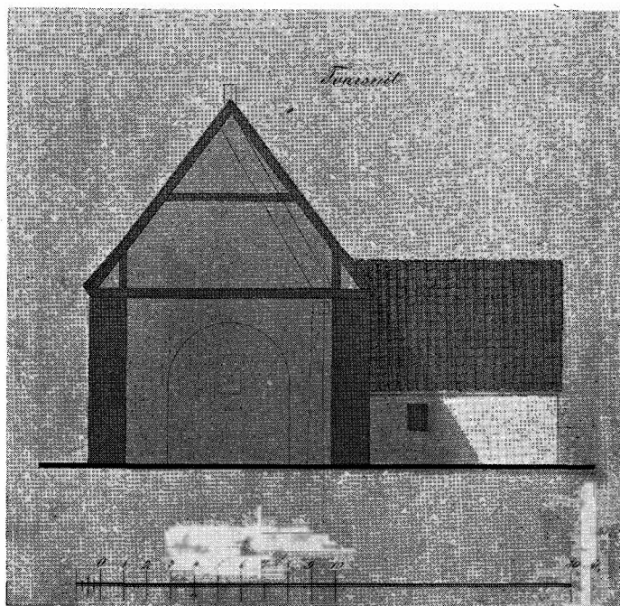
Uldum gamle Kirke, Tværsnit set fra Øst. Efter Tegn. i Nationalmuseet af Tage Olivarius.
