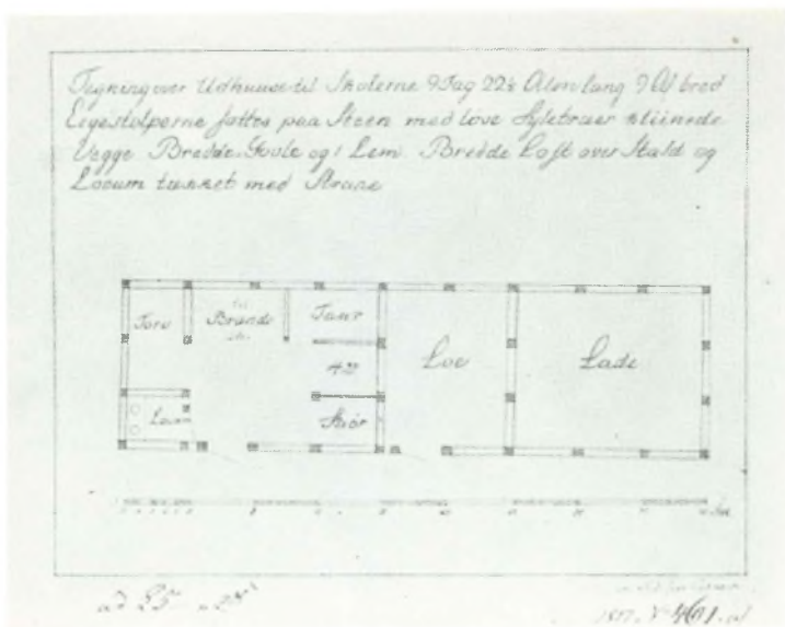
17. Standardtegnning fra 1817 til et udhus ved skolerne. (Rigsarkivet)
