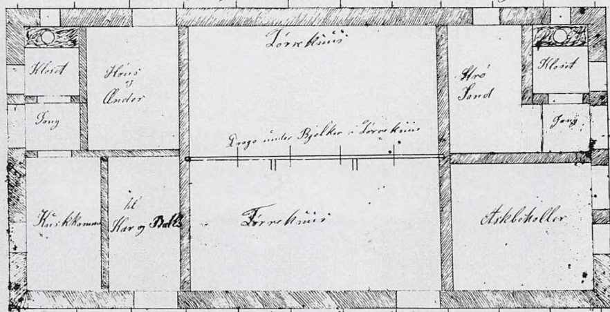
Grundtegning til en Løve Kæmpe paa 11 Alen
