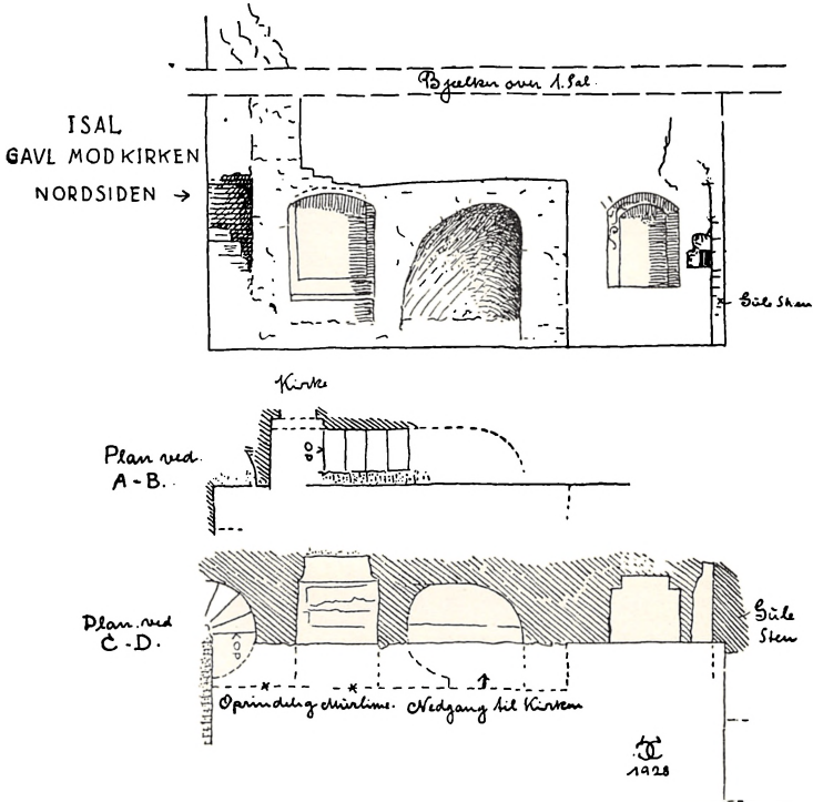
Fig. 5. Trappen til 1. Sal og Taarntrappen. Øverst: Gavlvæggen paa 1. Sal ind til Kirken. Plan af Trapper, Stue og 1. Sal. Maal 1:100.
