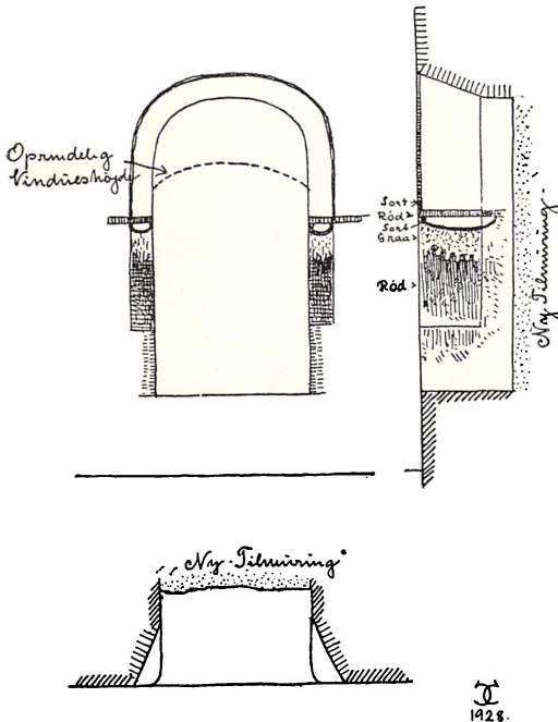
Fig. 8. Vindue paa 1. Sal i Vestmuren med malede Dekorationer fra Renæssancetiden. Maal 1:50.
