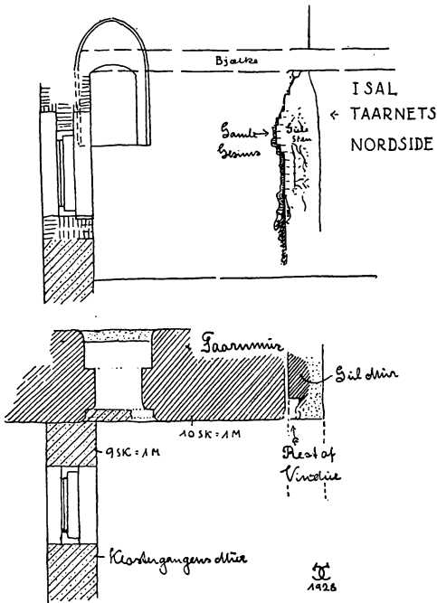
Fig. 2. Gl. Vindue i Taarnets Nordvæg. Maal 1:100.
