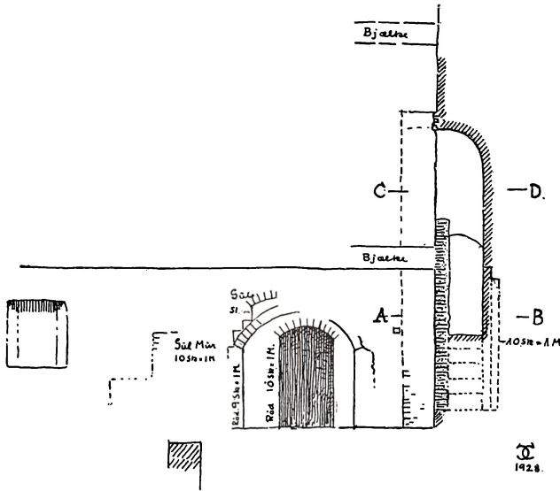
Fig 4. Snit af den gamle Trappe fra Stuen til 1. Sal. Paa Bagvæggen Dør ind til Taarnet. Maal 1:100.
