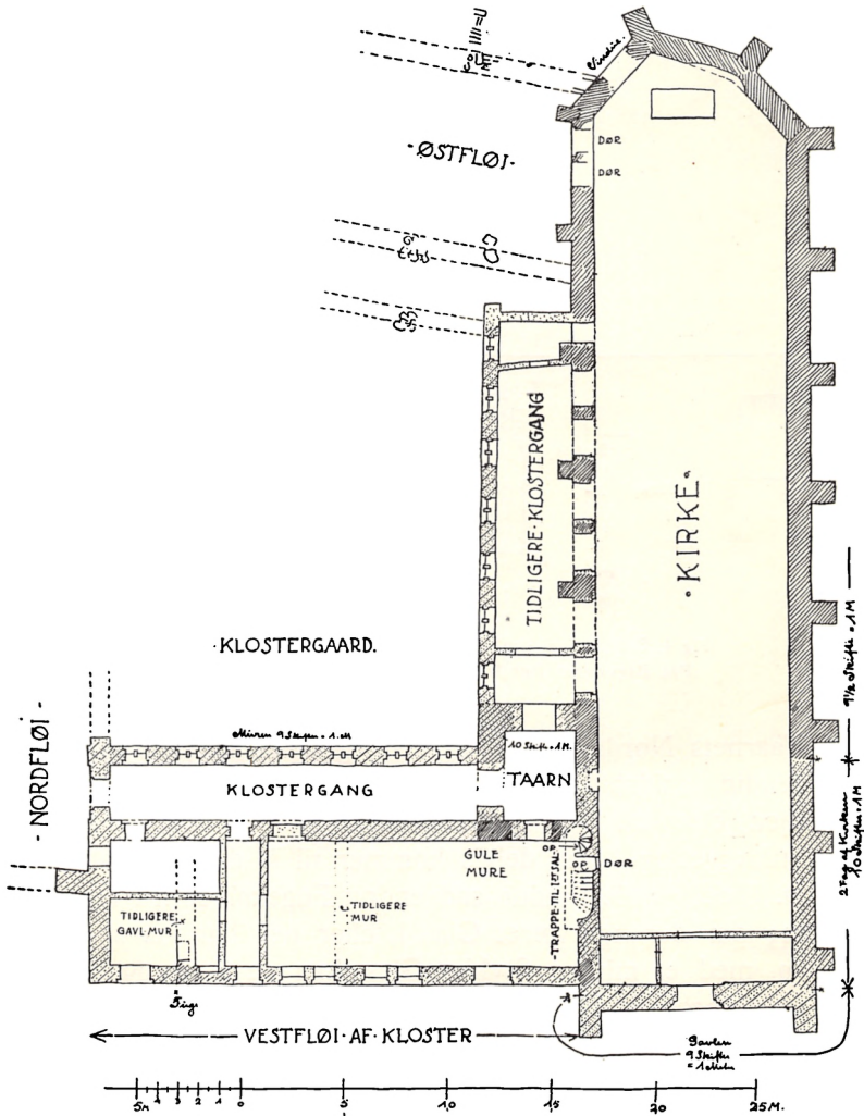
Fig. 3. Grundplan af Kirke og Kloster. Øst opad.
