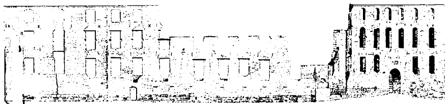
Koldinghus 1895. Opmåling af sydmuren udført af arkitekt Julius Smith på bestilling af baron Raben-Levetzau. Dele af sydmuren blev nedrevet 1881–84. Original tegning. Museet på Koldinghus.
