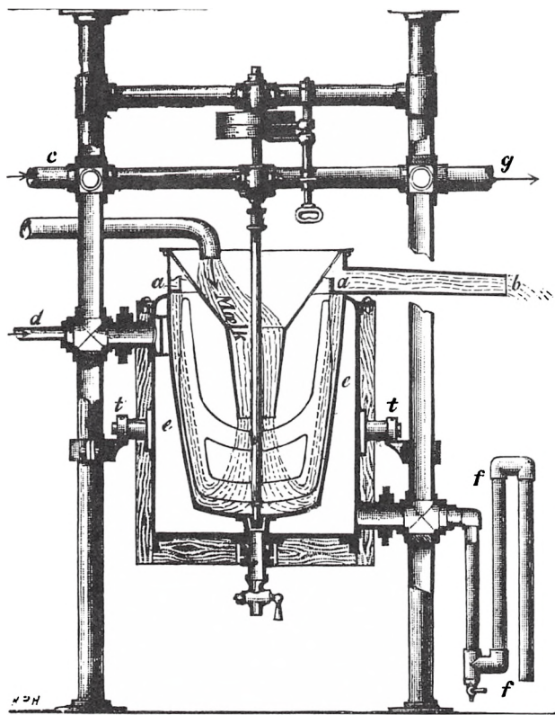
Skummetmælkspasteuriseringsapparat med paraboloidformet varmeflade.
