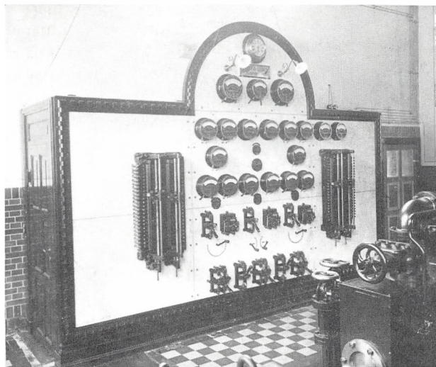
Værkets første tavleanlæg med instrumenter og afbrydere i midtersejlet. I sidefelterne ses celledskifterne til batteriet.
