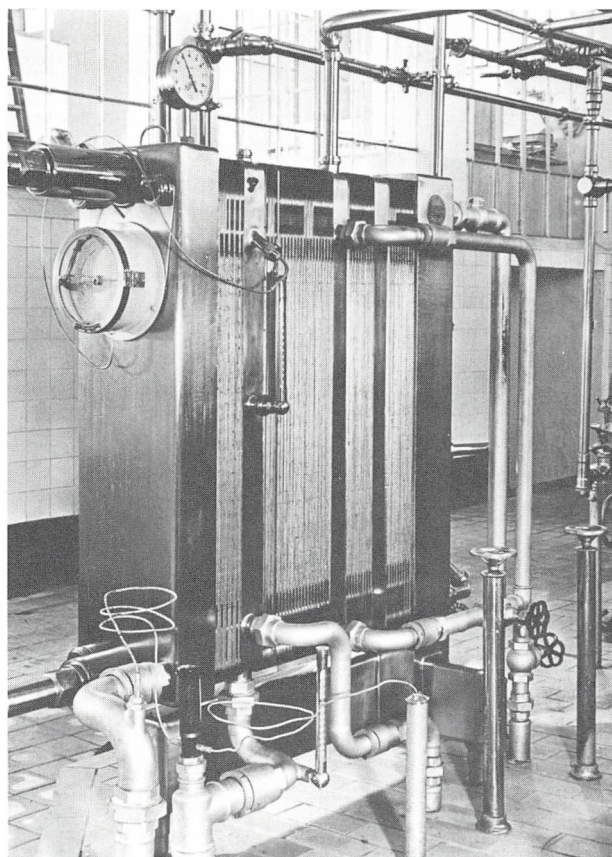
Pladeapparat type TK fra 1950. Dette apparat var DDMM's første egenkonstruktion efter krigen. Det var en presset plade med påsvejsede kantlister hvorimellem en 4 mm gummisnor dannede pakningen.
