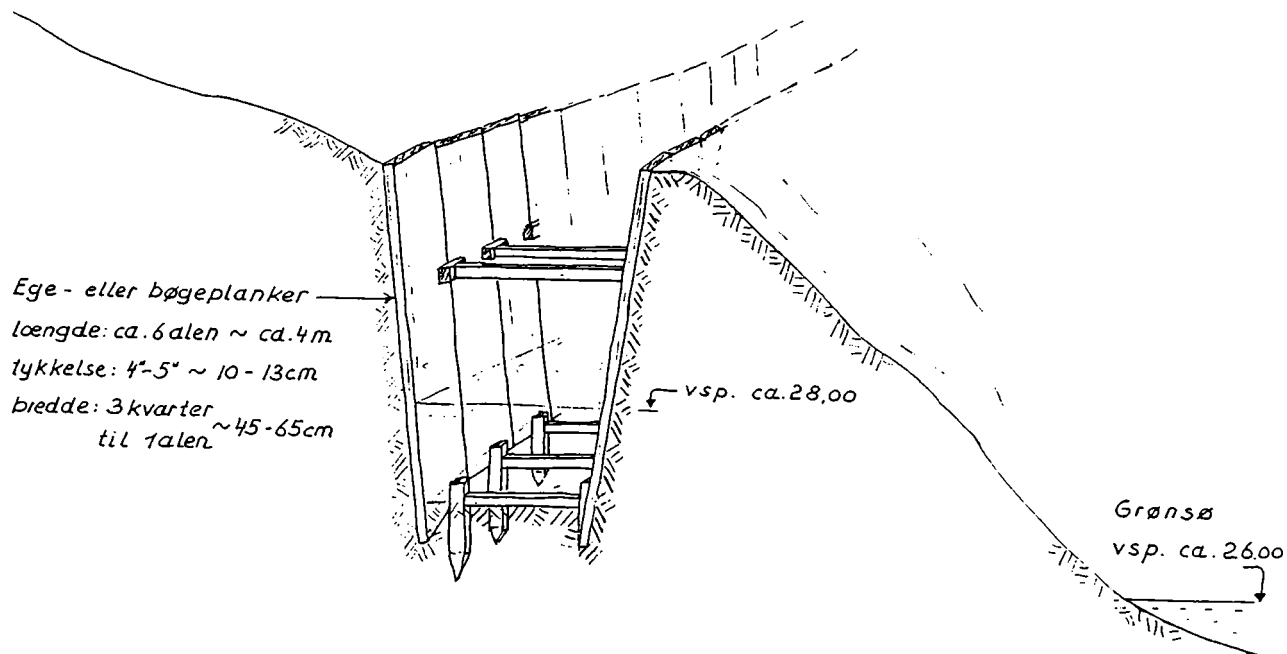
Tværsnit af kanalen »Saltgrøften« ud for Grønsøen.
