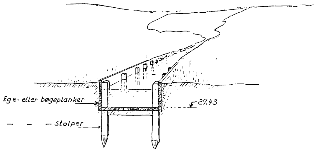
Tværsnit af kanalen »Saltgrøften« ca. 150 m syd for Stallerup sø.
