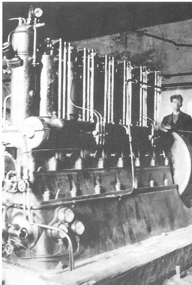
Binderup Elektricitetsværk dieselmotor. I baggrunden bestyrelsen.
