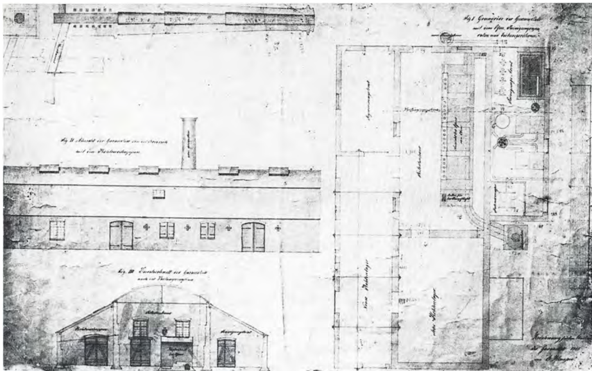
Grundplan og facadetegning af gasværket 1868, udarbejdet i forbindelse med indretning af lerretortet. Bygningen er den i 1857 af Paul Christiansen opførte.
