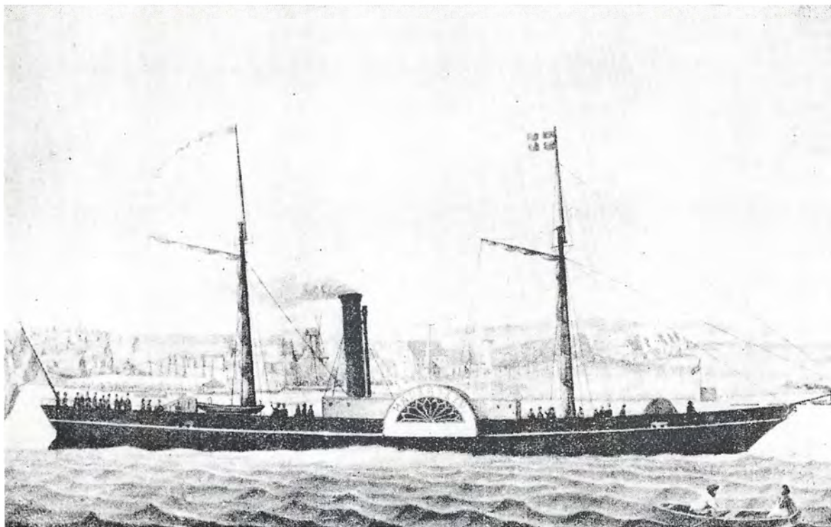
Ijuldampskibet Haderslev, bygget å Wolfgang Petersens jernstøberi g maskinfabrik 1859–60. Som det es var det tillige udstyret med sejl. baggrunden vind- og korndamp- nøllen ved havnen, til højre huse- angs den nuværende Lindedal.
