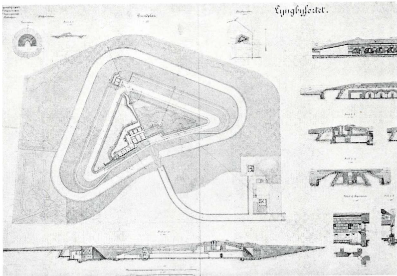
4. Plan over Lyngby Fort. Fortlegemets karakter af en retvinklet trekant ses tydeligt. Strubekasernens beliggenhed og vestre halvdel af kontraskarpe-kaponieren ses til venstre for den rette vinkels halveringslinje. Til højre for den ses fortets dæk med panserkuplernes placering. (Hærens Arkiv).
