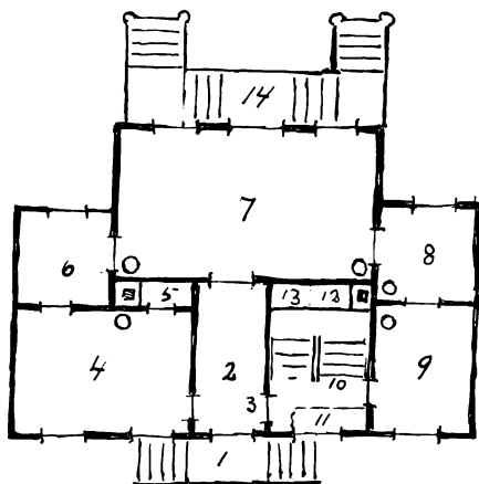
Rids over stueetagen. 1 Stentrappen, 2 Entré, 4 Spisestuen, 5 og 12-13 Skabe, 6 og 8 Kabinetter, 7 Havestuen, 9 Rygestuen, 10 Trappeopgang, 14 Havetrappen.
