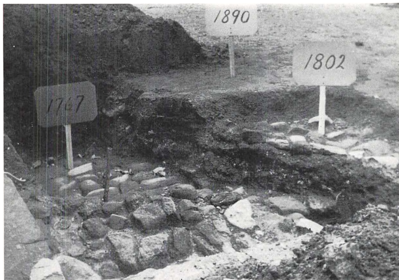
Afdækning af 3 gårddækninger. 1767 Brolægning fra Holmskjolds stald. 1802 Ramées brolægning. 1890 Carl Allers makadamisering.
