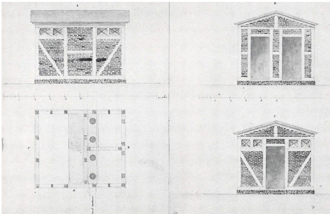
Ramée's tegning til udhus (opvaskerum og locum).
