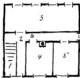
Rids over 2den sal. 1 Trappe, 2 Garderobe, 3 Carl Allers stue, 4-5 Værelser, 6 Garderobe, senere elevator.
