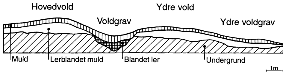
Lodret snit gennem dobbeltvolden i Halsted Dyrehave. Tegn.: Anette Krøyer.
