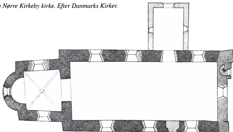
Grundplan Nørre Kirkeby kirke. Efter Danmarks Kirker.
