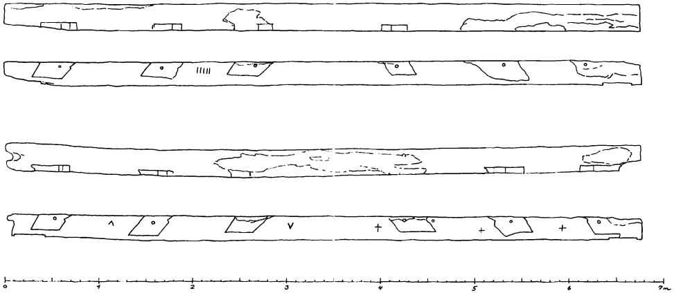
Opmåling af de to gavlbjælker fra klokkestokværket, plan og opstalt.
