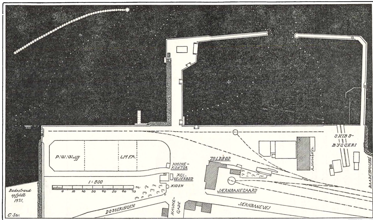
Fig. 11. Stubbekøbings tredie Havn efter 1911 samt den i 1931 byggede fjerde Havn Vest for. De Arealer i begge Bassiner, der ligger inden for de punkterede Linier, har en Vanddybde paa 6 m (Tegningen fra 1932).
