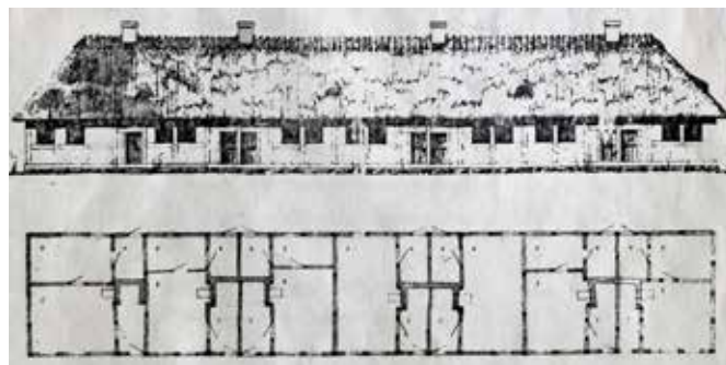
Plan og sydfacade af Greve Hospital på Frilandsmuseet. 1:200. Børge Erhardt.
