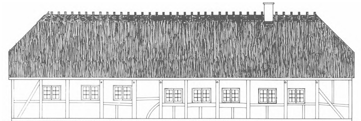
Standrids af østfacade (haveside)
