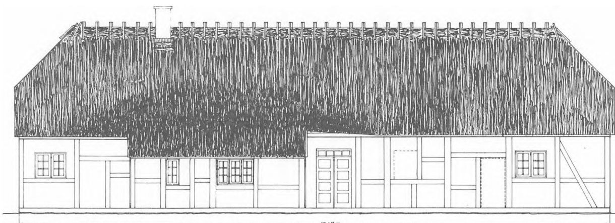
Standrids af vestfacade (gårdside)
