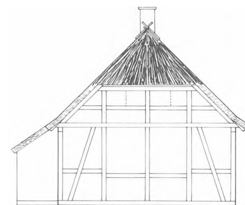
Standrids af sydgavl
