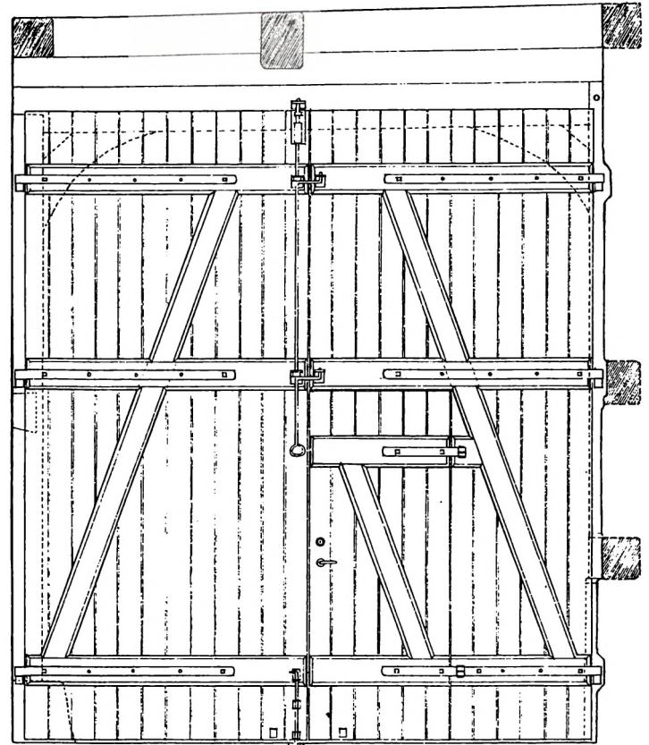
OPSTALT, SET FRA PORT-RUM
