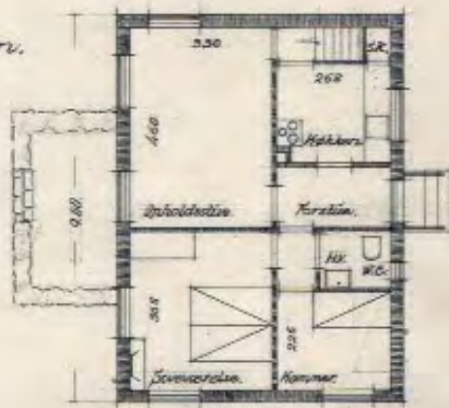
Stueplan.
