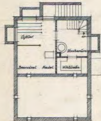
Kælderplan.
