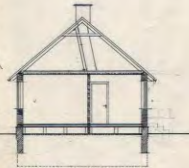
Tværsnit.
