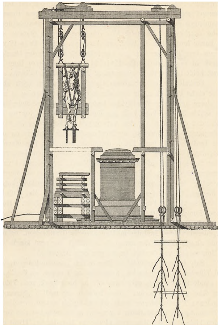
Maskineriet ved Rytterstatuens Opstilling.
