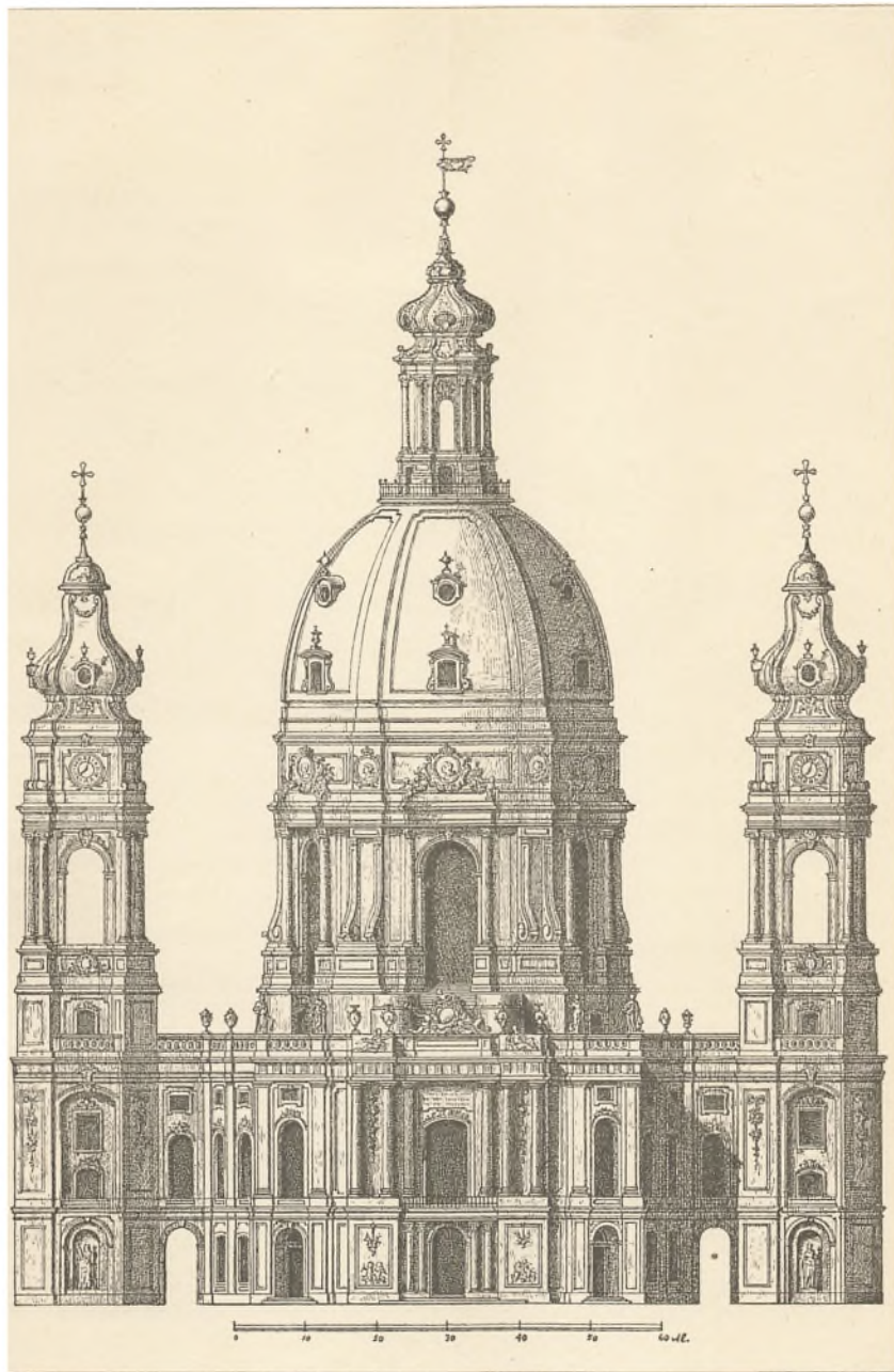
Eigtveds ændrede Udkast til Frederikskirken, dat. 10de April 1754. (Efter en i 1892 til Rigsarkivet afleveret Tegning.)
