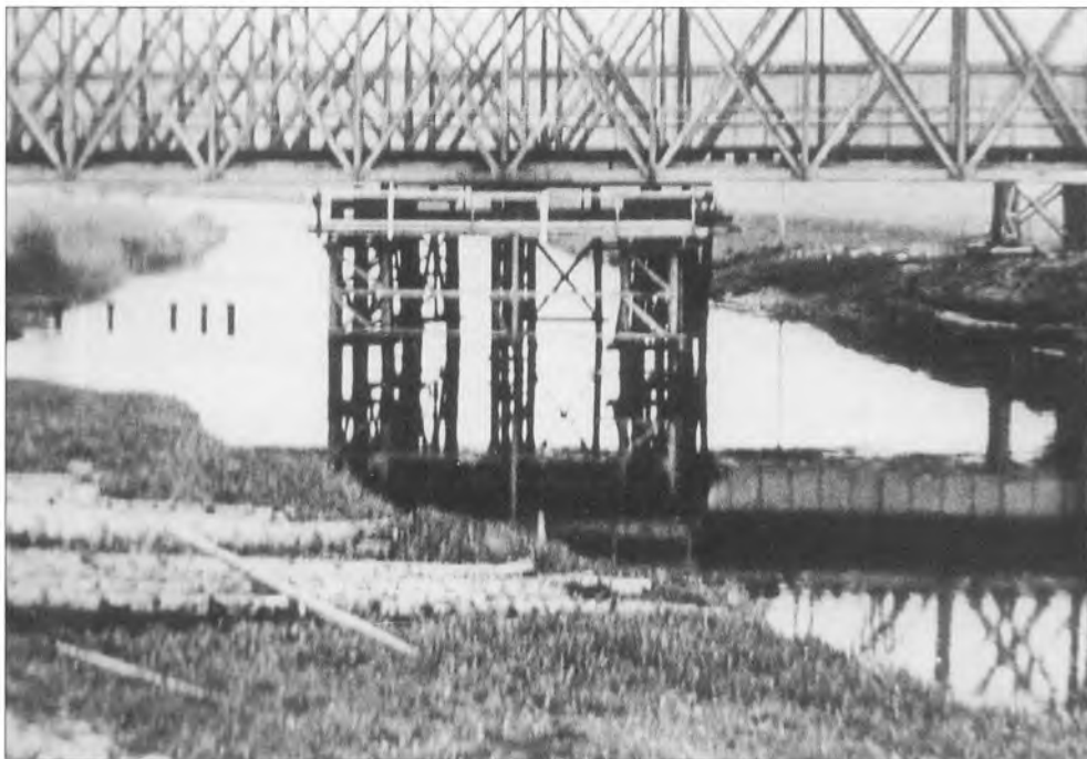
Gitterbroerne blev understøttet midt i Gudenåen. De kunne benyttes efter 11 dage.
