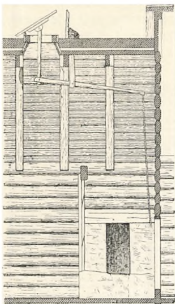
Fig. 25. Snit af Røgovnsstue fra Sandven, Vikør. Lyren aabnes ved leddelt Lyre-stang. (Efter „Kunst og Haandværk“.)
