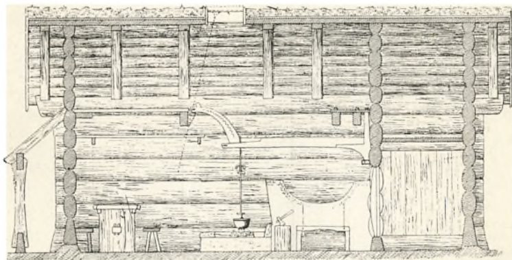
Fig. 30. Tværsnit af Fig. 29 Arnestuen paa Kvæstad, Valle i Sætersdalen. (Efter „Kunst og Haandværk“.)
