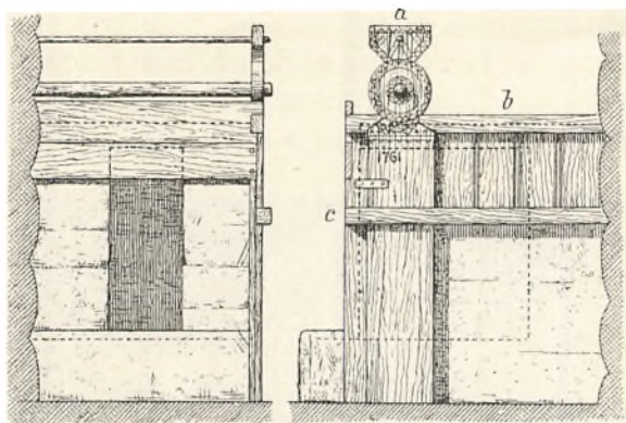
Fig. 33. Røgovn fra Opheim i Hardanger. Forside og Tværside. (Efter „Kunst og Haandværk“.)
