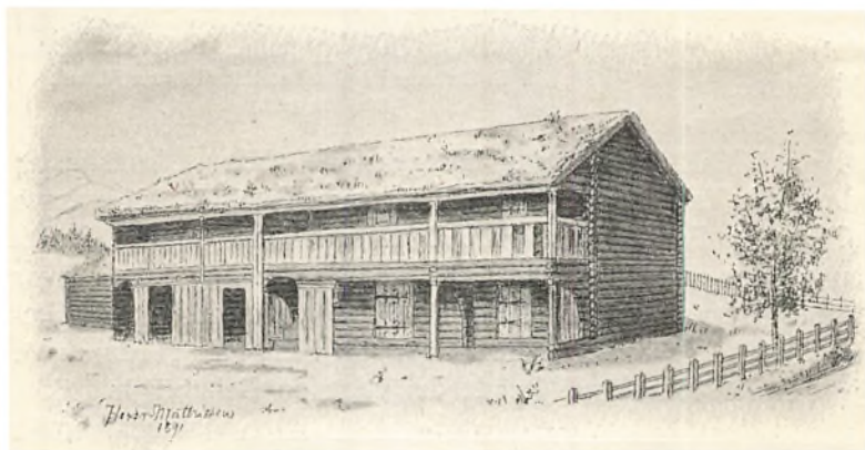
Fig. 78. Loftshus paa Ramsmoen, Tønset, Norge. (Tegning af Henrik Mathiesen 1891.)
