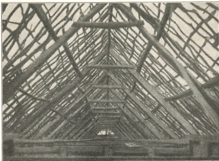
Fig. 13. Tagværket fra en Gaard paa Næs i Nørre Skaane, nu i Dansk Folkemuseums Frilandsafdeling ved Lyngby.
