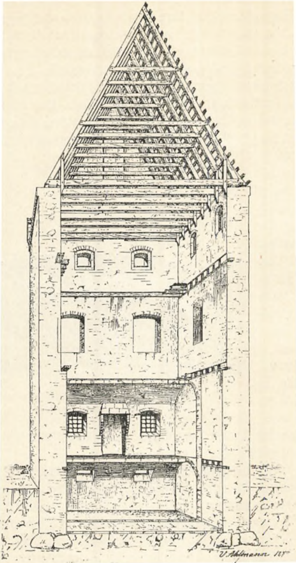
Fig. 131. Gennemsnit af Hovedbygningen paa Vedbygaard (Sjælland). (Tegnet af V. Ahlmann.)
