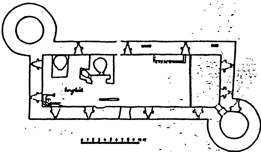
Lyckå slott. Markvåningen.
