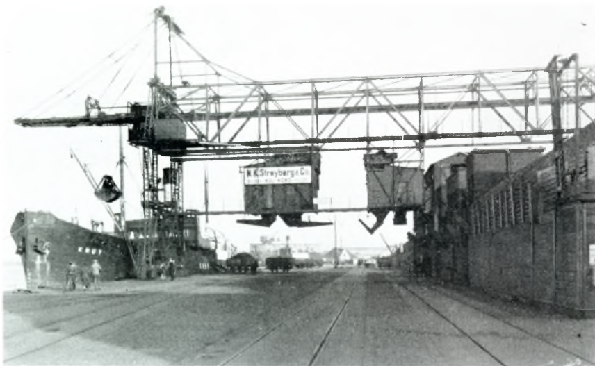
N. K. STROYBERG & CO.'S KRAN- OG UDLEVERINGSANLÆG
