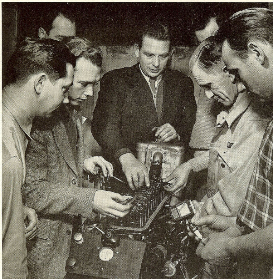
Læreren i motorlære, B. Henriksen, viser sine elever, hvordan kompressionen måles. Til venstre står Sigfred Mortensen, P. Rasmussen og Svend Jensen — og på den højre side af Henriksen skimtes B. Bahr, mens Tage Hjort står med kompressionsmåleren i hånden og Knud Jensen holder et tændrør.
