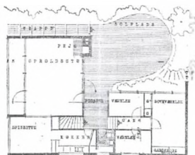
PLAN AF ØVERSTE ETAGE
