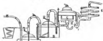
Fig. 3. Brændevinsapparat med smekkeskiver, eller Friedrichs Gøring. Beskrivelse over Bøe, del 4 og 5, side 4, dele 1 og 2, side 3.
