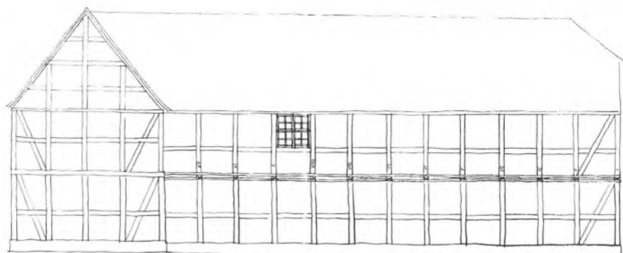
STENGADE 63, HELSINGØR, OMKRING 1750; GAVL SAMT SIDEHUS UD TIL SANKT ANNA GADE. REKONSTRUKTIONSFORSØG, 3/4-1998 /JKJ
