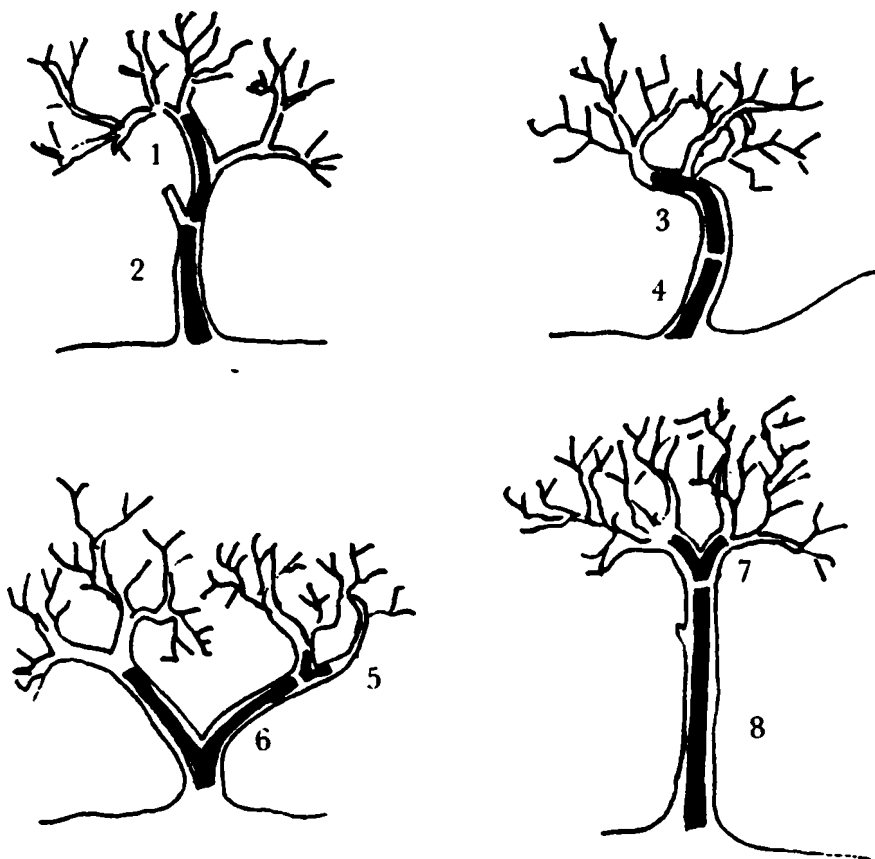
Tommerdele der kan fremelskes fra træerne er unge. 1. topspant, 2. bundspant, 3. kranbjælke, 4. sitters (ovre spantedel), 5. alm. knæ. 6. underste hækbjælke, 7. skarp bundstok, 8. agterstævn. Efter R. G. Albion: Forests and Seapower (1926).
