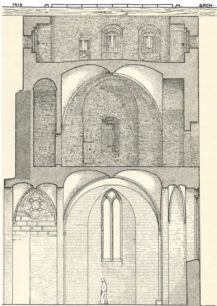
Fig. 5. Køge Kirketårn. Reconstr. Snit, Øst-Vest, gennem tre nedre Stokværk.
