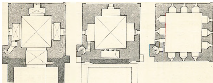
Fig. 2-4. Reconstr. Planer af Køgetårnets tre nedre Stokværk i deres Tilknytning til Gammelkirken. (Opm. Cl.-H).
