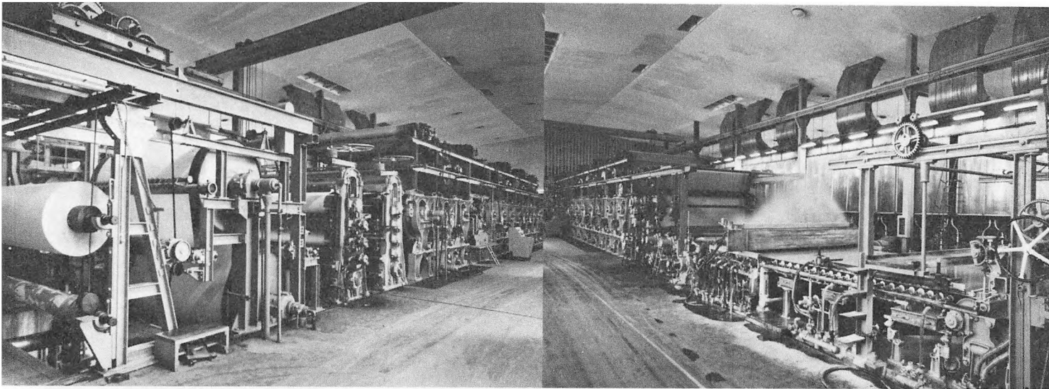
SPI's bestyrelse orienterer sig for tiden om køb af en af de brugte papirmaskiner, der kan fås i Europa og USA. — Her er den, hvorom opmærksomheden har samlet sig — fotograferet dels fra den ene ende og dels fra den anden. Maskinen er ca. 70 m lang og ca. 10 m høj. Ca. \frac{1}{3} af maskinens højde ligger under gulvet. Vægten er ca. 375 tons.
