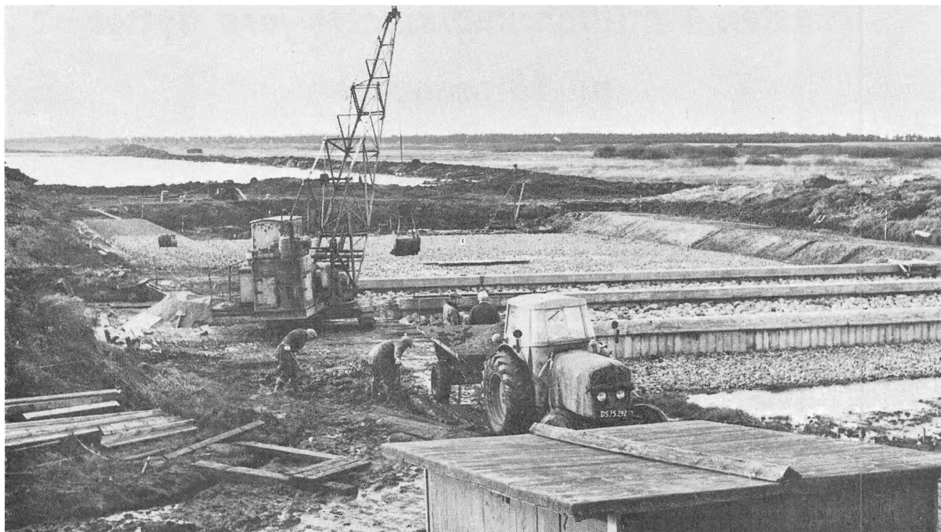
Et kig ud over arbejdspladsen ved Kodbøl, hvor et 65 meter langt styrt og Nordens største fisketrappe bygges. I baggrunden til venstre det nye åløb.
