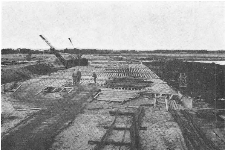
Den nye hovedvejsbro bygges »tørskoet«. Her et kig ud over den nye, brede vejbro.
