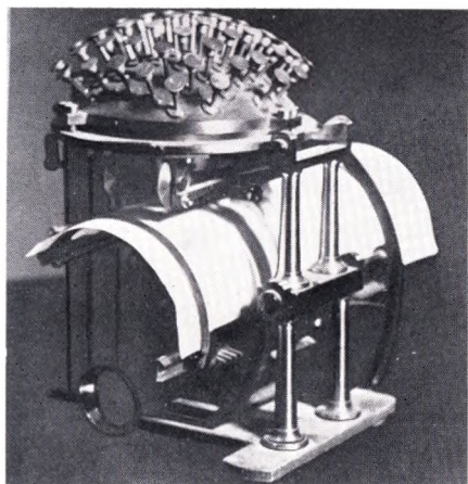
Danskeren Malling-Hansen fik Eneret paa sin Skrivekugle i 1870.
