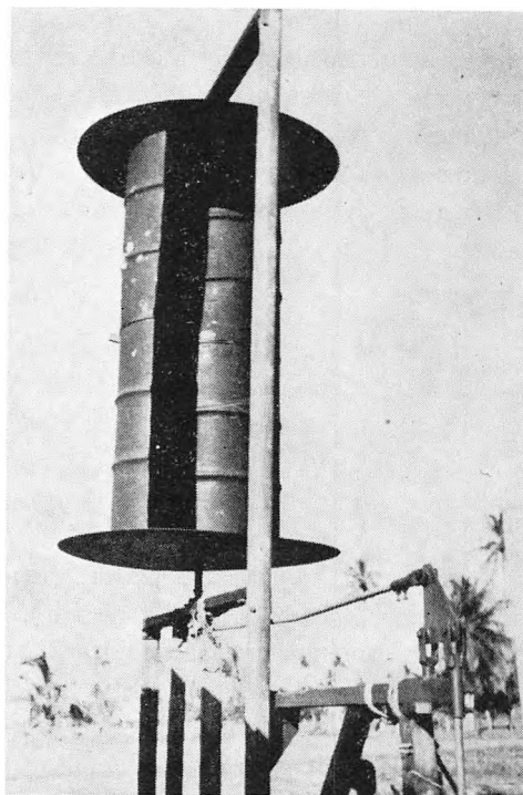
Fig. 6. Vindmølle lavet af to overskårne olietromler. Denne mølle anvendes til pumpe på Ceylon. Meget billig og simpel at konstruere.
