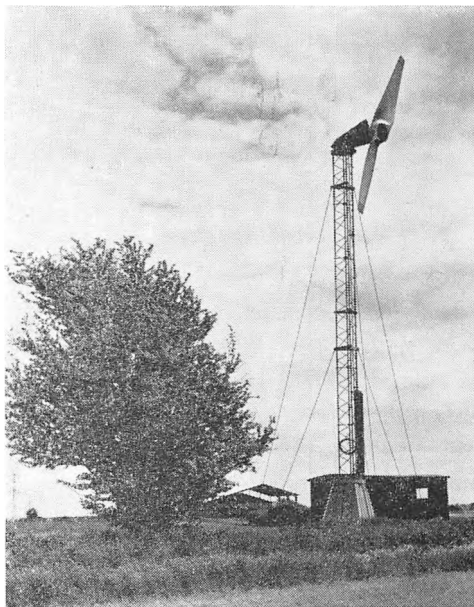
Fig. 1. Varmemølle fungerende efter vandbremse-systemet, Jordbrugsteknisk Institut, KVL, Maskinhal, Vridsløsemaglevej 19, Tåstrup (se note 2).
