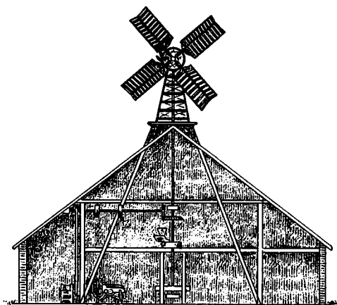
Klapsejlsmølle. Afbildet ca. 1900 i katalog fra T. C. Nielsens maskinfabrikker, Hjørring.
