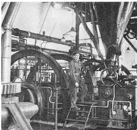
Et hjørne af maskinhallen i den store briketfabrik i Pindstrup. Herfra sendtes per døgn gennem mange år 120 tons tørve- eller brunkulsbriketter ud til danske kækkeovne og fyr.
