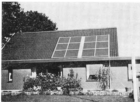
Fig. 7. Solfang installeret i villatag efter næsten samme princip som ved solfangeren fig. 5. Opvarmer brugsvand og vand til svømmebassin. Installeret af Per Alling, Kabelvej 5, V. Hassing Strand, Vodskov.
