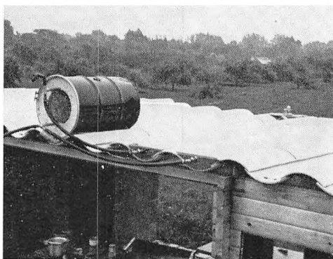
Fig. 5. Simpel solvandvarmer. Består af to solfangere indbygget i et tag. Solfangerne er via plastic-rør i forbindelse med isoleret beholder, hér udført af lille olietromle inden i større. Solfangerne består af isolering nederst, sort metalplade med indlagt rør i midten og ét lag glas øverst. Gennem glasset opfanges solvarmen, der p. g. a. isoleringen kun kan »slippe ud« via vandet, der i dette system vil være 40—50° varmt ved 16—17 tiden. Bygget af forfatteren i sommeren 1973 på eksperimenthuset på Brace Research Institute i Montreal. Princippet anvendes i dag flere steder i Danmark og har været i anvendelse i Israel, USA og Australien i meget lang tid.
