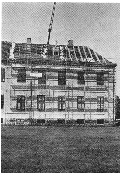
Moderne kran letter taglægningen ved restaureringen af Clausholm. 17. juni 1974.
