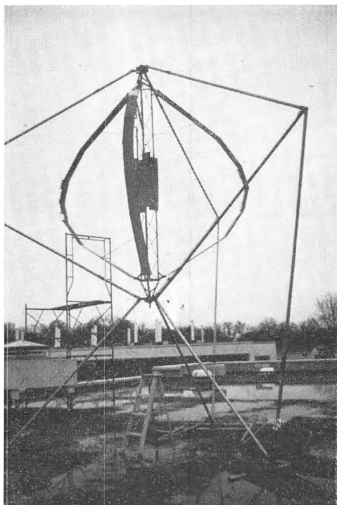
Fig. 3. Darrieux-rotor med en diameter på 4,3 m. Drejer om en lodret akse. Der eksperimenteres flere steder med denne mølle, f. eks. indgår den i de hollandske Fokkerfabrikkers planer om en eventuel vindmølleproduktion. Møllen hævdes at have en meget stor ydelse pr. anvendt kg metal. Billede fra: National Science and Research Council, Ottawa.
