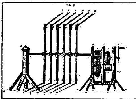
Festers tærskemaskine. Omkring 1760 konstruerede Didric Fester en maskine med 6 roterende dobbelte plejle, som kunne trækkes med hånd- eller bestekraft.
