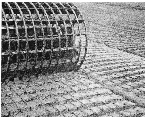
Når den opgravede tørvjord har været gennem ælteværket, køres »grøden« på tipvogne ud på læggepladsen. Her formes massen til tørv af den store, hestetrukne formetromle.
