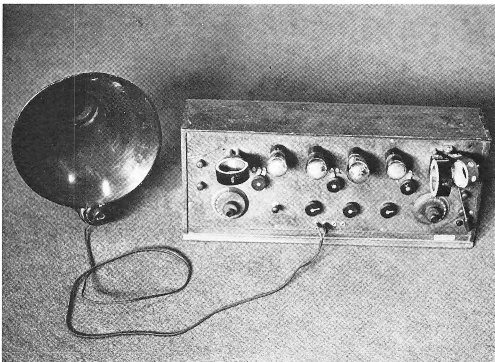
Denne radio, som tilhører Lokalhistorisk Samling i Hammel, er fra 1920'erne. Den oprindelige ejer var montør Marius Nielsen, Hammel, som brugte den indtil ca. 1960. Fot.: S. P. Andreasen, Farre, 1975.
