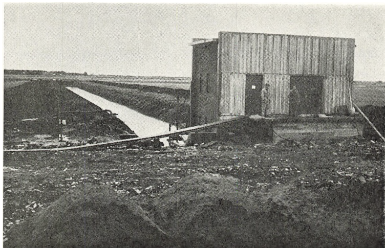
Pumpestation »Ø« i Damsø har en kapacitet på 2000 liter vand pr. sekund.
