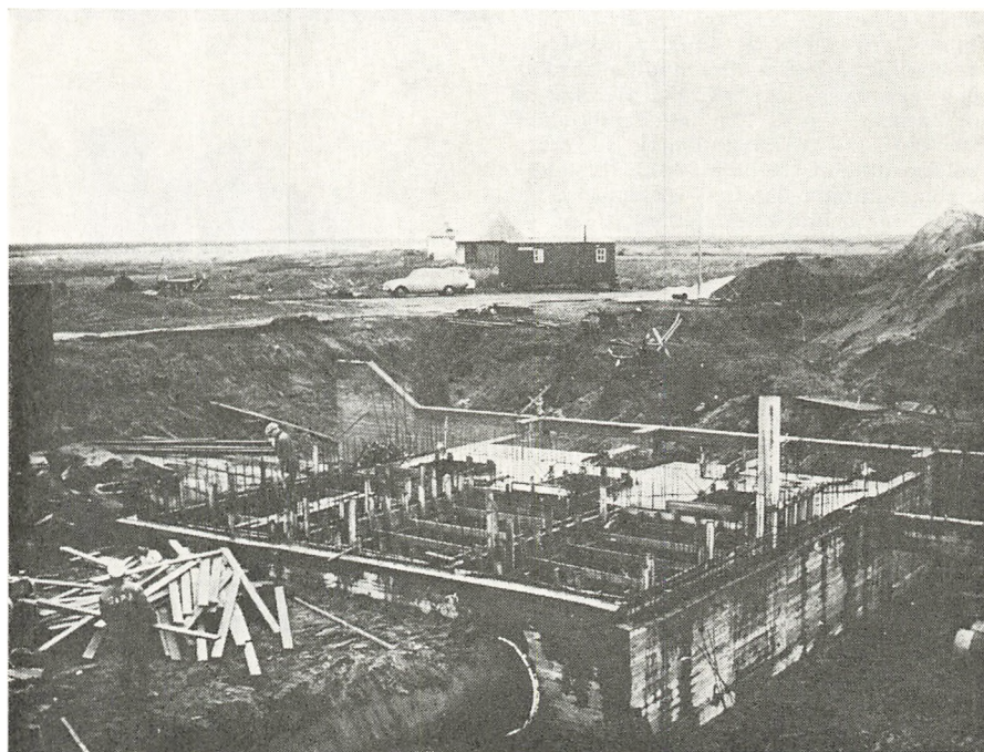
Billedet herover viser byggepladsen ved »Proustgaards« hus ved Nyå og Blindå mellem Skjern og Stauning. I forgrunden det underjordiske fundament til projektets største bygværk, pumpestation »Nord«, der rejses i 2½ etages højde.
