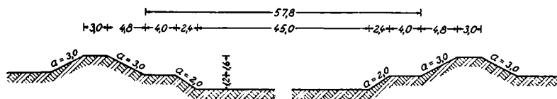
Ovenstående viser det udarbejdede projekt omkring Skjern å. Til højre vises profil af åen med diger.
