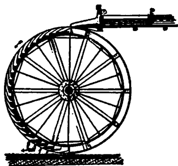
Overfaldshjul.
