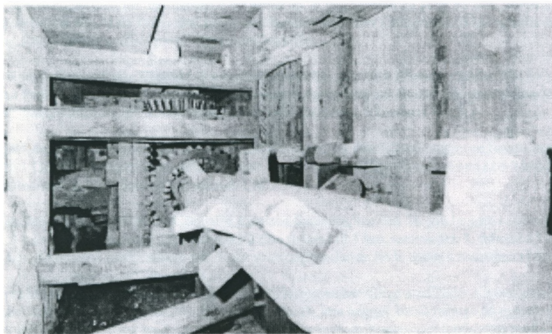
Stampværkets vandrette aksel med stampeløfterne
