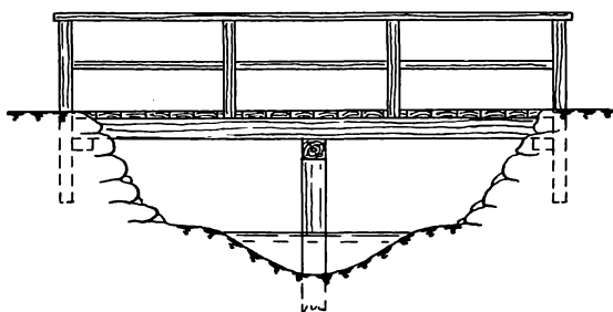
Rekonstruktionsskitse af Stilling Dams Bro. Standrids.
