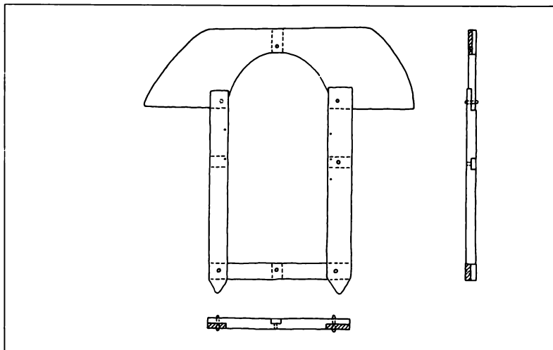
Fig. 6. Egetræskarm fra romansk vindue. Mål 1:20. Øverst t.v. opstalt, t.h. lodret snit, nederst vandret snit. Overkarmen er punktvist rekonstrueret efter aftryk i mørtelen.
