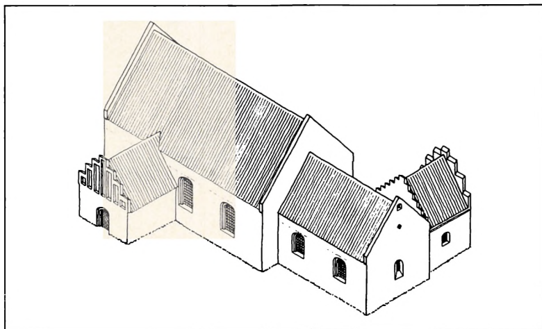
Fig. 21. Skib og kor forhøjes og hvælv indbygges. Taggavlene afsluttes med museastråpning. Sakristi i teglsten med selvstændige kamtakkeede gavle tilbygges korets nordside. Sengotiske vinduer.
