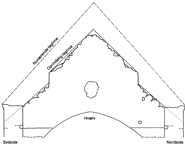
Fig. 26. Skibets vestgavl set fra tagrummet. Mål 1:100.
