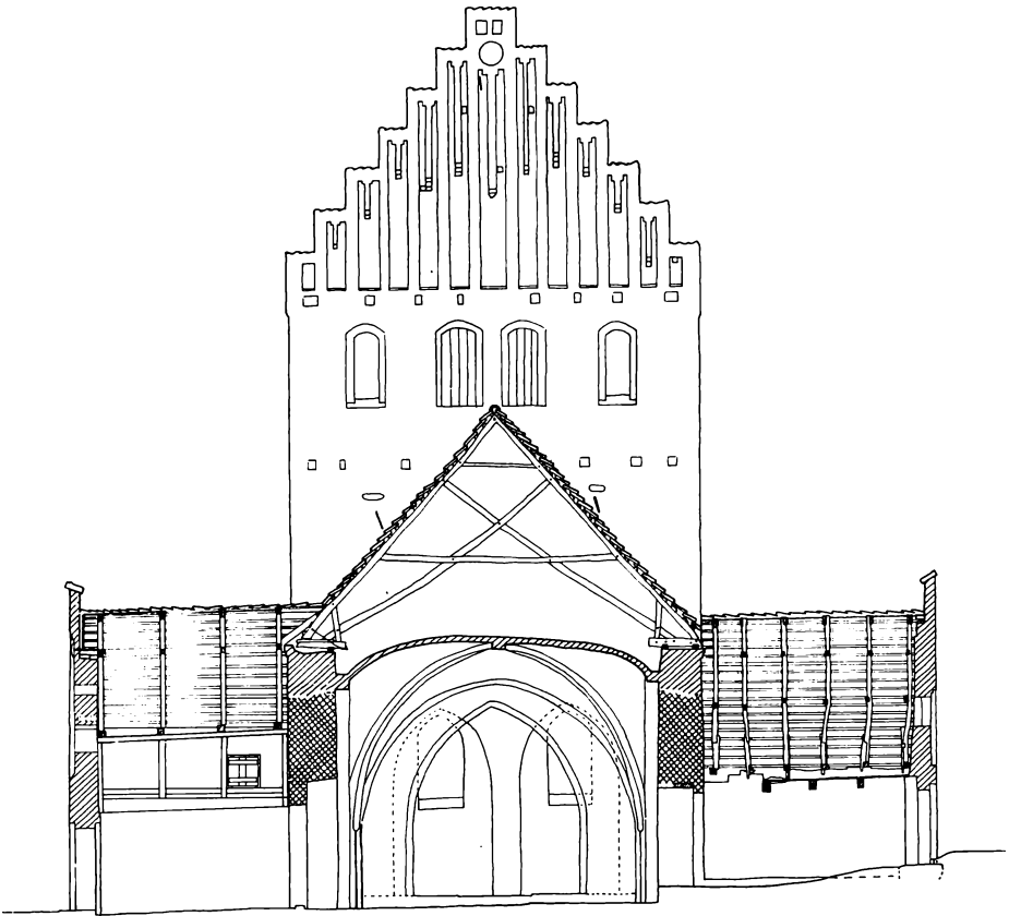
Fig. 4. Snit gennem søndre våbenhus – skib – nordre våbenhus. Mål 1:200.
