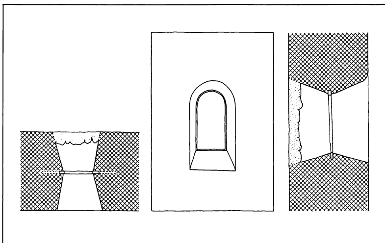
Fig. 7. Romansk frådstensvindue. Mål 1:50. T.v. vandret snit, i midten opstalt, t.h. lodret snit. På snittene ses den nyere tilmuring ind mod skibet.
