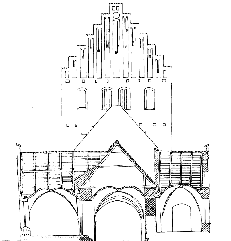
Fig. 5. Snit gennem gravkapel – kor – sakristi. Mål 1:200.
