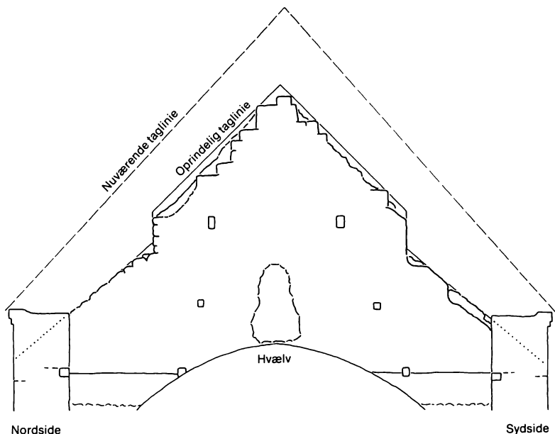
Fig. 25. Triumfgavlens vestside. Mål 1:100.
