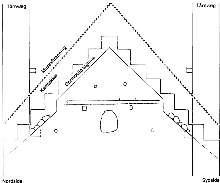
Fig. 27. Skibets vestgavl set fra tårnrummet. Mål 1:100. Tagafslutningens tre foregående faser. I feltet under den oprindelige taglinie ses øverst spor af 2 bombuller fra opmuringsstilladset; herunder spor af en trækbjælke fra et tidligere spærtæg.
