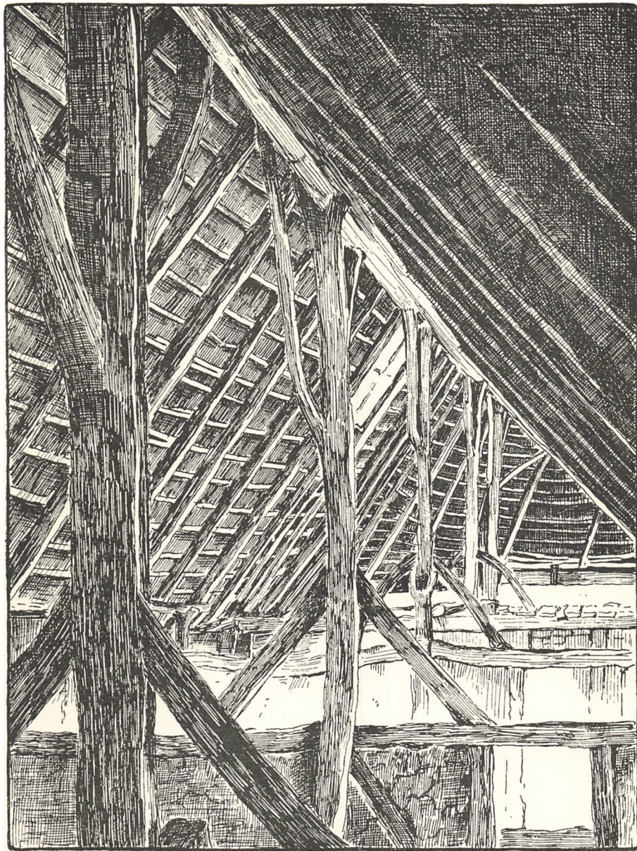
SKYDEBJERG PRÆSTEGAARD, ODENSE AMT BAAG HERRED
