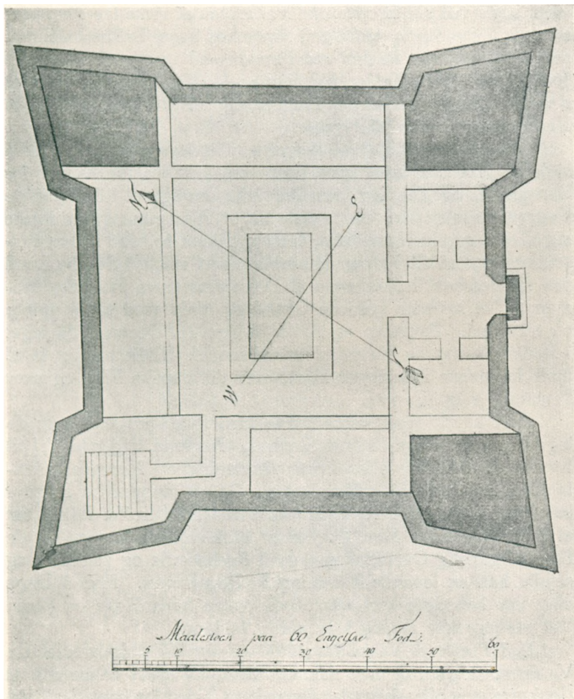
Grundrids af Fortet Augustenborg.
